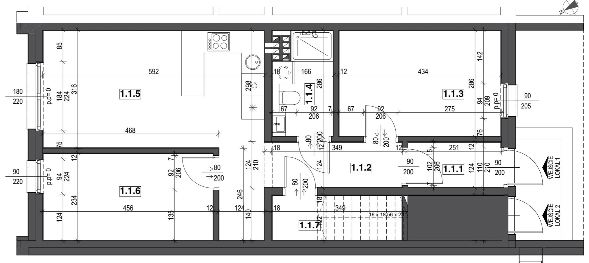
RZUT PARTERU
